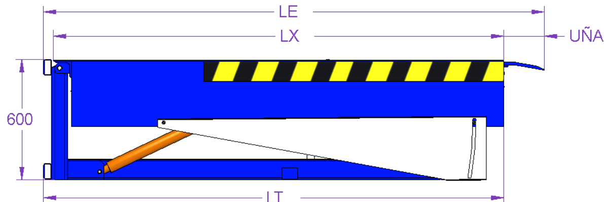
VISTA LATERAL SIDE VIEW VUE LATÉRALE
